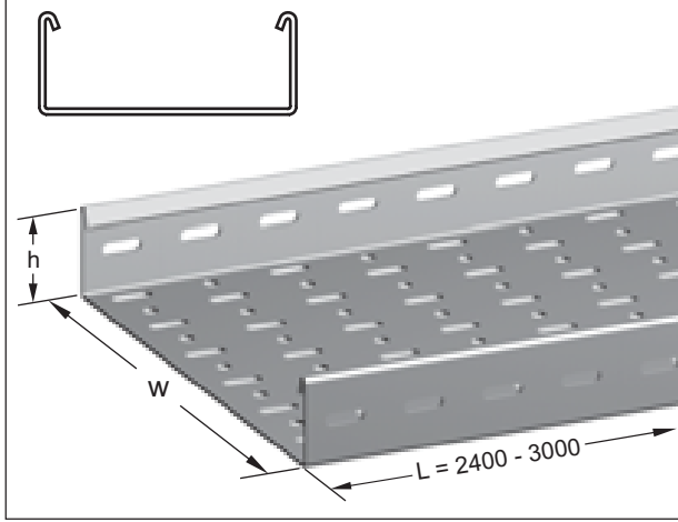
Cable tray perforated (Heavy duty design.) Delikli kablo kanalı (Ağır hizmet tipi)
