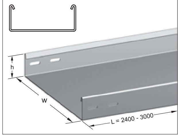
Cable tray unperforated (Heavy duty design.) Deliksiz kablo kanalı (Ağır hizmet tipi)
