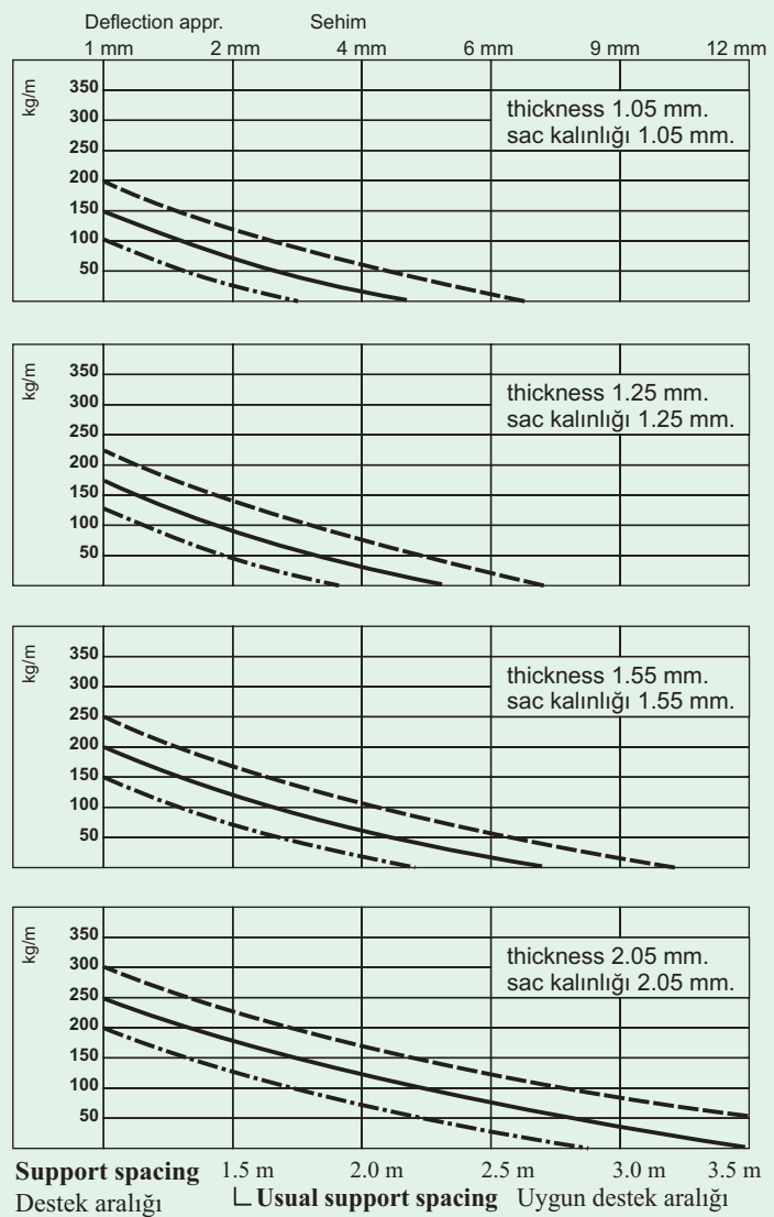
Diagrammes of loads for 4T 4-5-6 Yük diyagramları 4T 4-5-6 kanallar içindir
